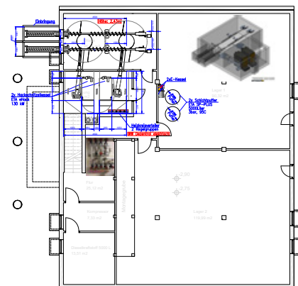
Bauhof: Grundriss UG mit 2 x Hackschnitzelheizung Text / Bilder: Ingenieurbüro Schötz
